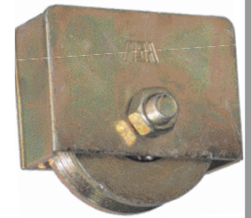
Rueda Maquinada con Caja 2" x ¾" cap. 72 kg 2 ½" x ¾" cap. 80 kg 3" x ¾" cap. 125 kg 3 ½" x ¾" cap. 150 kg
