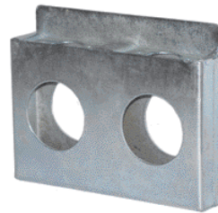
Porta Chapa embutido doble 1" calibre 14 1 ¼" calibre 14
